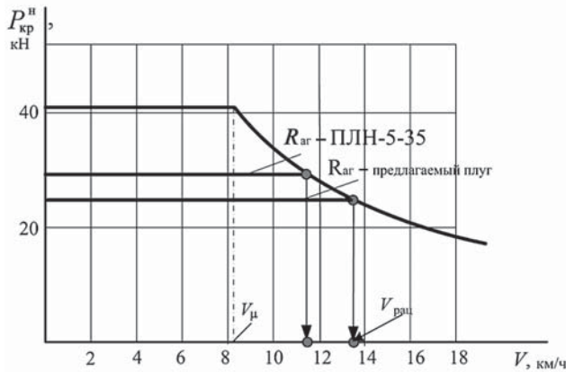
Рис. 2 – Потенциальная тяговая характеристика трактора К-3180
