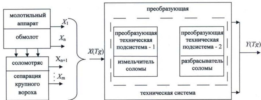
Рис. 3 – Структурная модель измельчителя-разбрасывателя соломы как преобразующей технической подсистемы зерноуборочного комбайна
